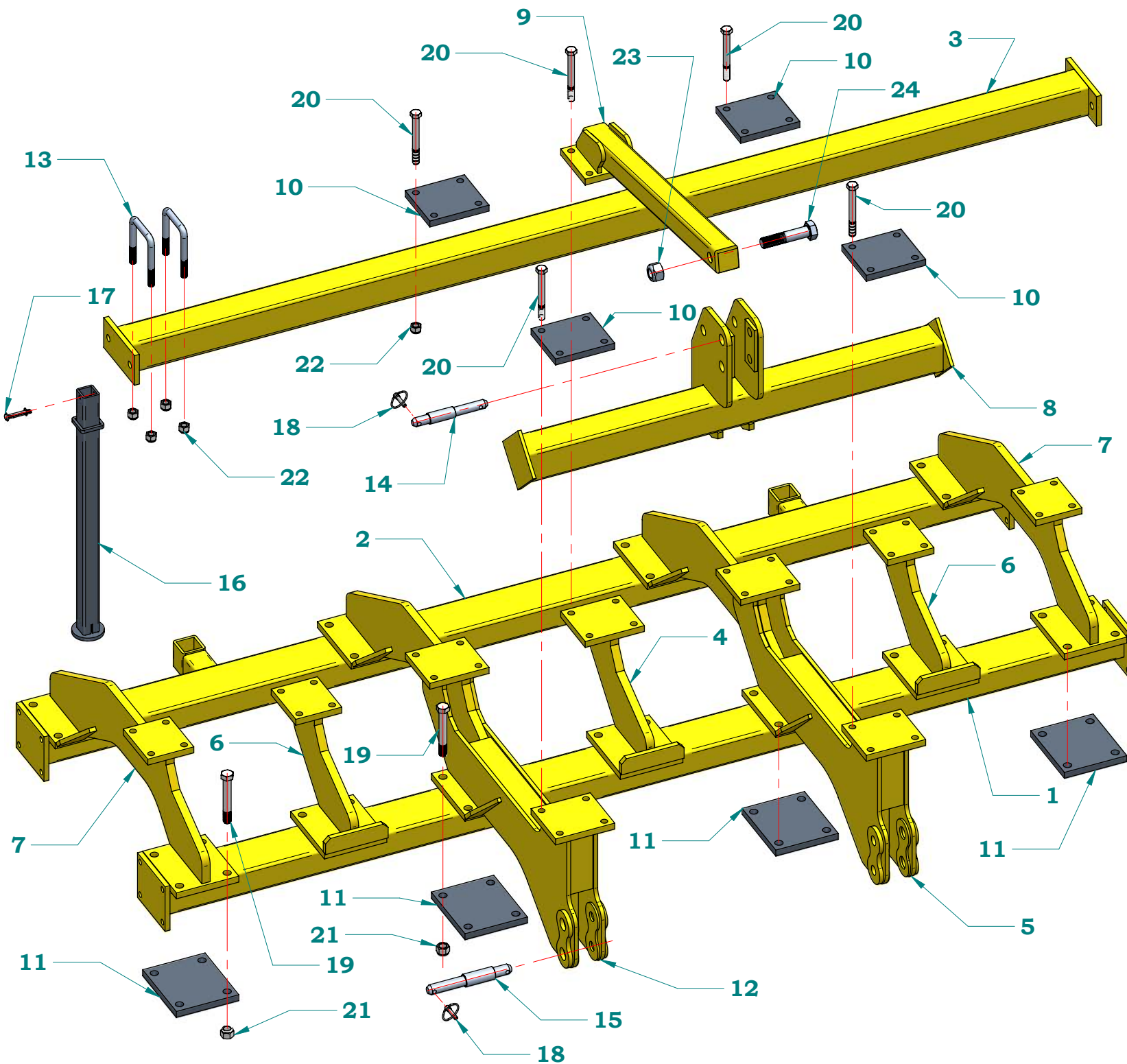
TAVOLA 1 RIPUNTATORE 707
